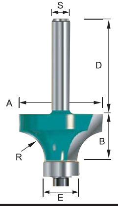
圆角刀 (带轴承)
