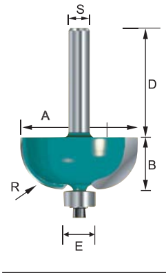
倒角刀 (带轴承)
