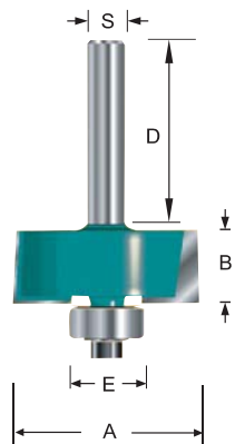
T 型刀 (带轴承)
